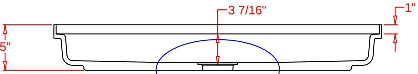
SECTION A-A
